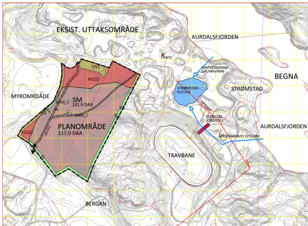
Fig.8 Illustrasjonen viser partier med løsmasser der vann fra Aurdalsfjorden trenger inn gjennom løsmassene og påvirker vannivået i Strømstadputten og ellers grunnvannsnivået i løsmasseforekomstene innenfor planområdet
