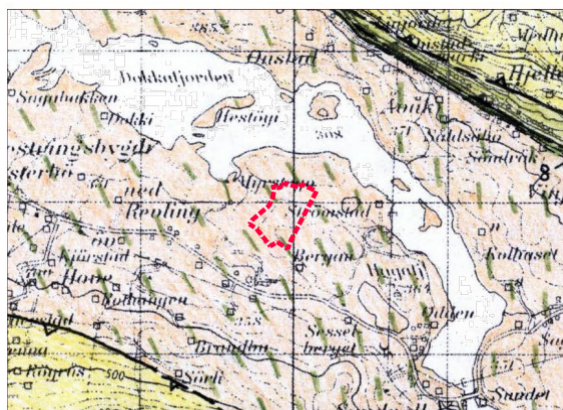
Fig.4 Gneis, båndet, grå til mørkegrå, med varierende kornstørrelse og til dels høyt kvartsinnhold; omdannet sandstein og skifer. Inneholder amfibolitt som flere steder er granatførende. Hovedbergarten er glimmerskifer.
