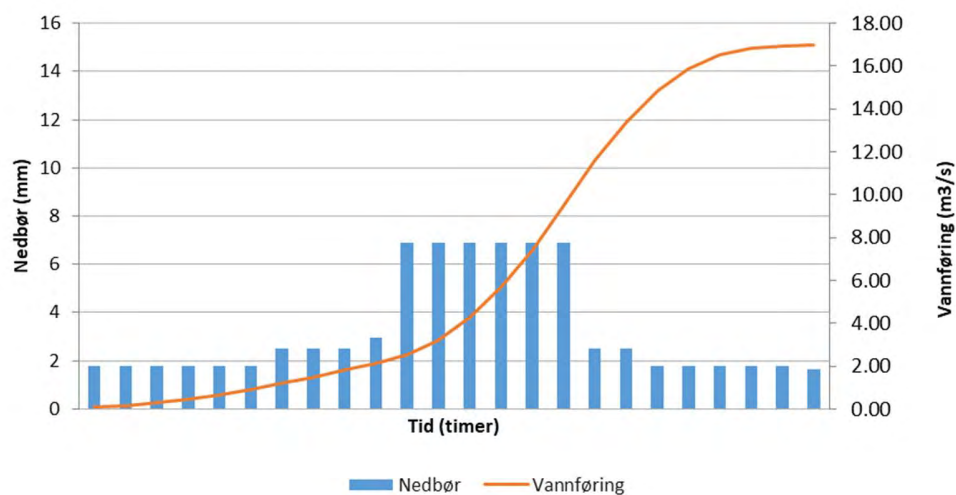
Figur 4.7. Nedbørforløp og beregnet kulminert 200-årsflom i PQRUT for effektiv sjøprosent lik 0,6%.
