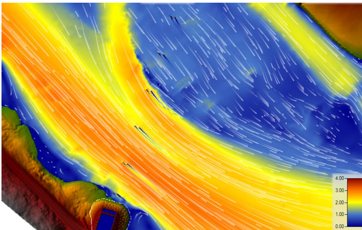
Figur 5-33. Vannhastighet og strømningsretninger omkring justert løsning med kassebru ved Q_{200} i Lågen og middelflom i Mjøsa (blå farge viser lave hastigheter, mens rød/ oransje farge høye hastigheter).
