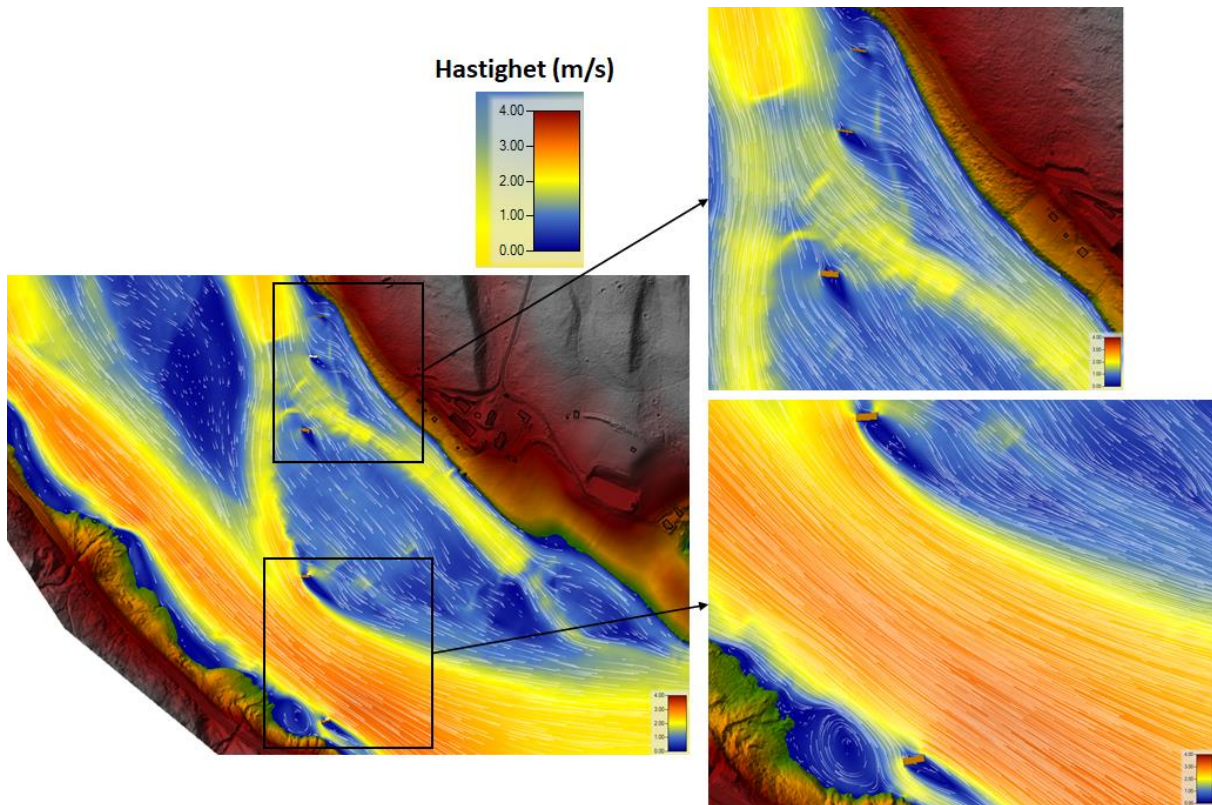
Figur 5-40. Vannhastighet og strømningsretninger omkring KDP-bru ved Q_{200} i Lågen og middelflom i Mjøsa (blå farge viser lave hastigheter, mens rød/ oransje farge høye hastigheter).
