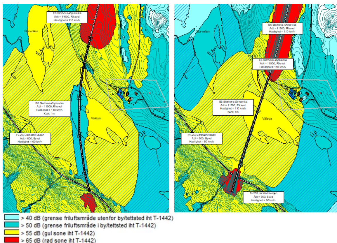
Figur 5-36. Beregnet støy fra trafikk på bruene for KDP-linjen (venstre) og justert løsning (høyre).
