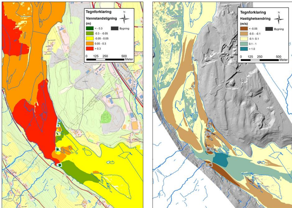
Figur 6-2. Simulering av vannstands- og hastighetsendringer ved Q_{20} i elva og middelflom i Mjøsa som følge av pilarer til KDP-bru, midlertidige fyllinger inkludert en 20 m lang bru nord for og 13 kulverter ute på Våløya.
