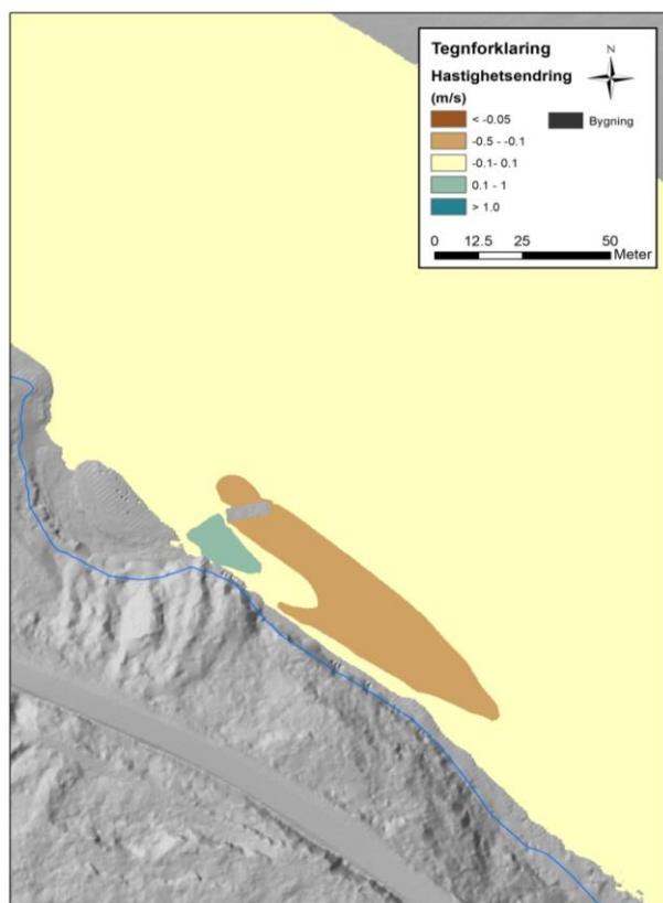
Figur 5-38. Simulering av vannhastighetsending ved Qmiddel i elva og LRV i Mjøsa for KDP-linjen med fritt frembyggbru. Bildet til høyre fremstiller utsnitt av detaljer omkring fundamentene
