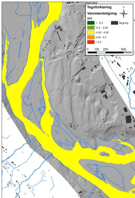
Figur 5-37. Simulering ved Qmiddel i elva og LRV i Mjøsa for Kommundelplanlinjen med fritt frembygg-bru viser ingen merkbar vannstandsending.
