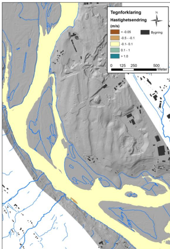
Figur 5-38. Simulering av vannhastighetsending ved Qmiddel i elva og LRV i Mjøsa for KDP-linjen med fritt frembyggbru. Bildet til høyre fremstiller utsnitt av detaljer omkring fundamentene
