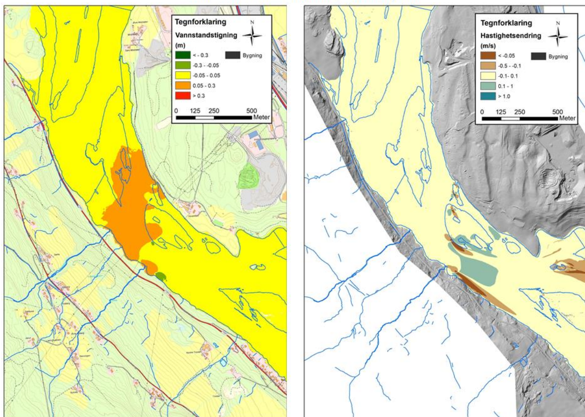
Figur 5-39. Simulering av vannstands- og hastighetsendringer ved Q_{200} i elva og middelflom i Mjøsa som følge av KDP-bru sammenliknet med dagens situasjon.
