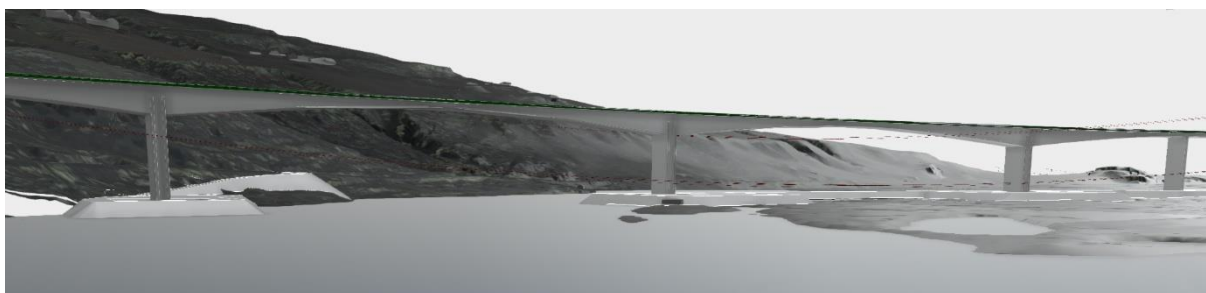
Figur 5-41. Denne bruløsningen gjør at den laveste av de eksisterende 300 kV-ledningene blir hengende farlig til midt i frihøyden under brua. Den øverste ledningen må legges om og det forutsettes at denne kan legges i samme høyde med brua.
