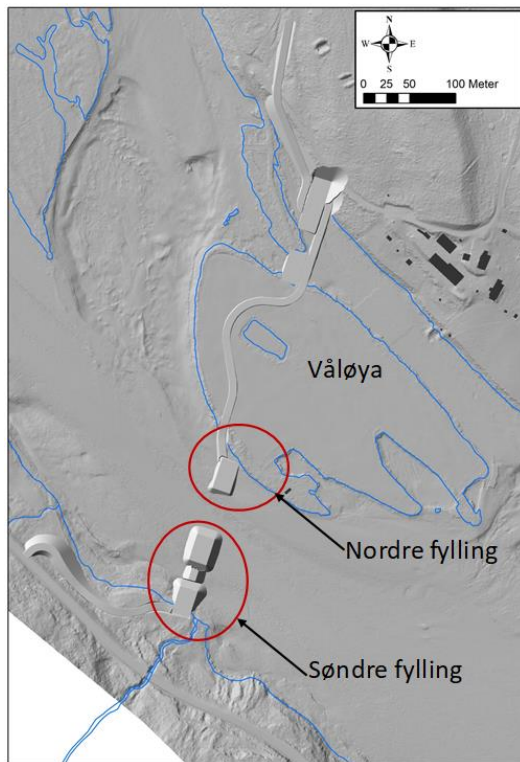
Figur 6-4. Planlagte fyllinger i anleggsfase for justert løsning med kassebru. Fyllingen i nord behøver ikke å være etablert samtidig som fyllingene i sør.
