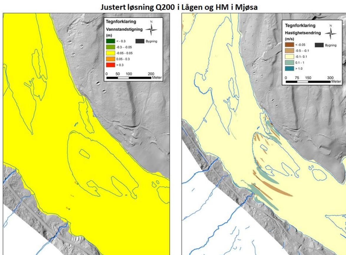
Figur 5-32. Simulering av vannstands- og hastighetsendringer ved Q 200 i elva og middelflom i Mjøsa som følge av pilarer til kassebru langs justert løsning.
