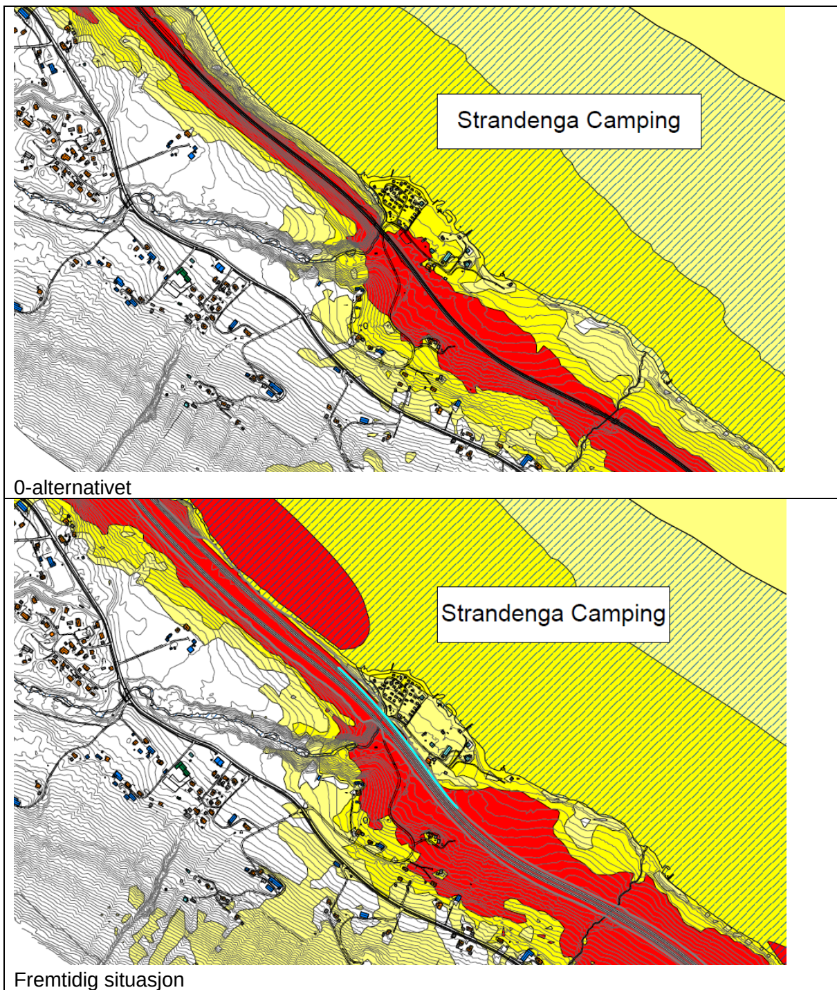
Figur 30: Støyberegninger langs området ved Strandenga Camping nord for Biristrand. Støysoner beregnet 1,5 m over terreng for å vise skjermingseffekt. 0-alternativet øverst, og fremtidig situasjon med støyskjerming i turkise linje nederst.
