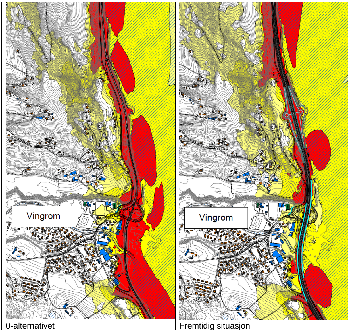
Figur 33: Støyberegninger ved Vingrom. Støysoner beregnet 1,5 m over terreng for å vise skjermingseffekt. 0-alternativet til venstre, og fremtidig situasjon med støyskjerming i turkise linjer til høyre.
