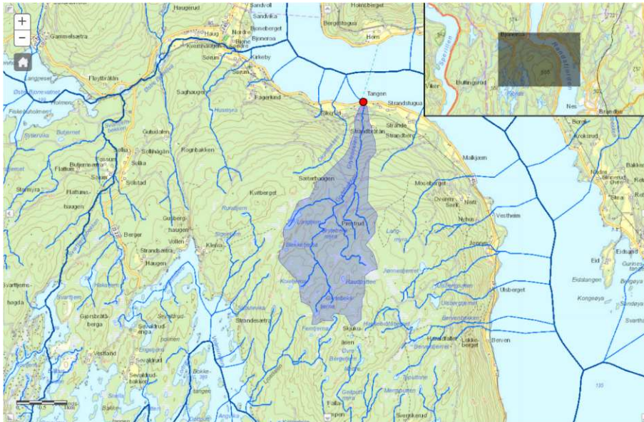
Figur 2. Nedbørsfeltet til Grytebekken, beregnet med kartverktøyet NEVINA. Utløpsoset ved fergekaia på Tange er merket av med rød sirkel (kilde NEVINA). Se flere detaljer i eget vedlegg.
